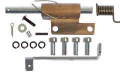
ITEM# 33369 HINGE PIN KIT
