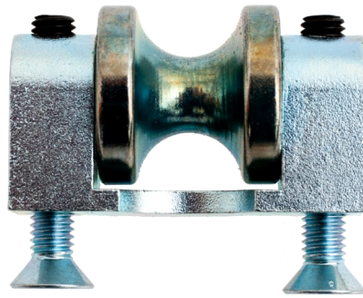
ROLLER STRAND KIT - C2/C p/n 33393
