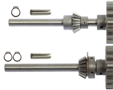
ITEM# 35481 R.H. / L.H. PINION ASSEMBLY
