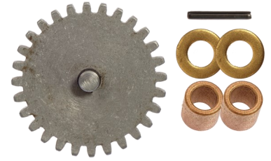
Idler Gear & Shaft Kit - J2/C2/C p/n 33274
