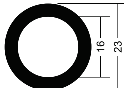
89558 18 mm tube
