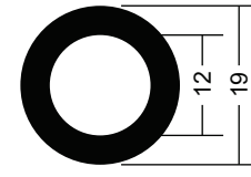
89555 14 mm tube
